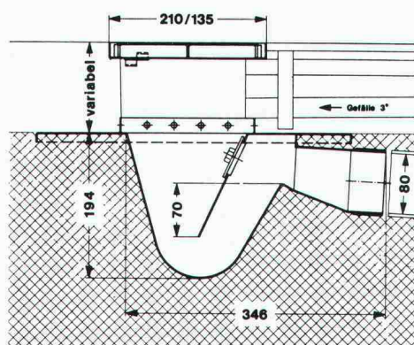
Bodenwasserablauf NW 80
