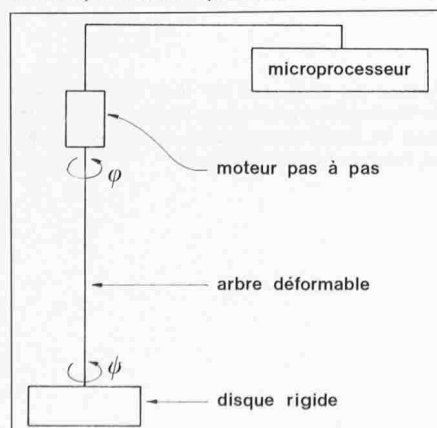
Figure 1. Un pendule de torsion actionné à son extrémité supérieure par un moteur pas à pas commandé au moyen d'un microprocesseur
