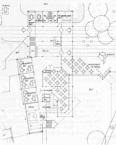
Grundriss Erdgeschoss 1: 900
