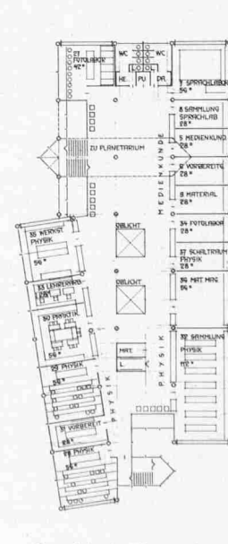
Grundriss 2. Obergeschoss 1: 900
