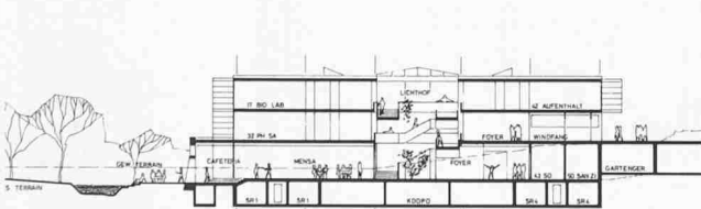
Schnitt 1: 900
