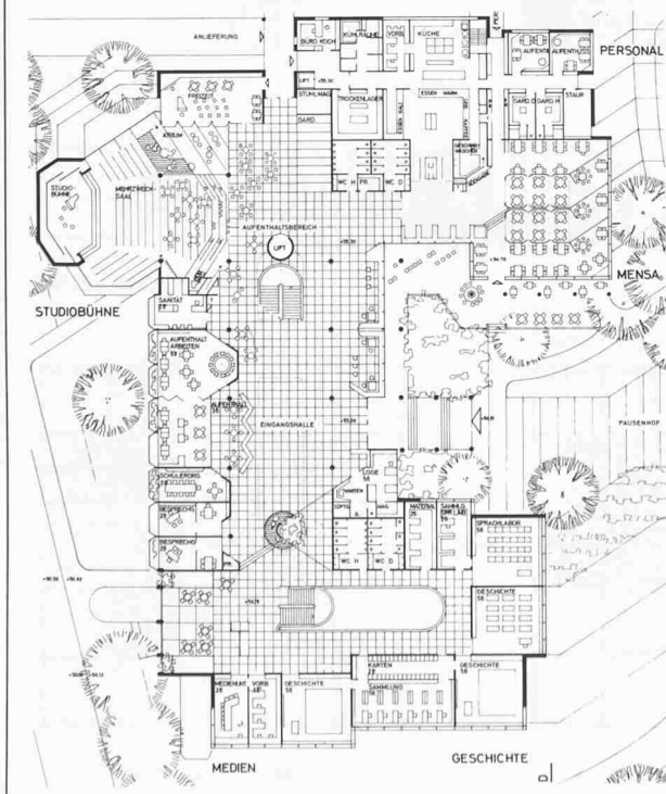
Grundriss Erdgeschoss 1:900
