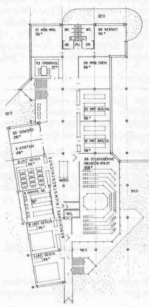
Grundriss Untergeschoss 1: 900
