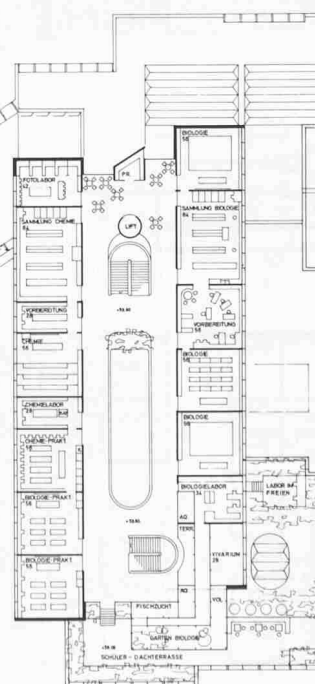
Grundriss Obergeschoss 1:900
