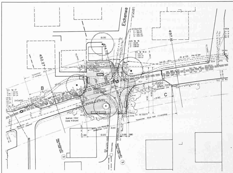
Wohnstrasse: Detailplan der Platzgestaltung
