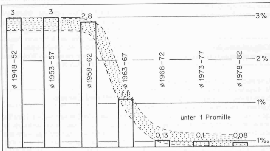
Bild 2. Staubauswurf in Prozenten der Produktion
