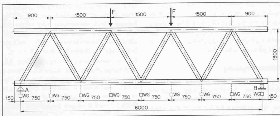
Bild 3. System, generelle Abmessungen und Kräfteinleitung der untersuchten Träger
