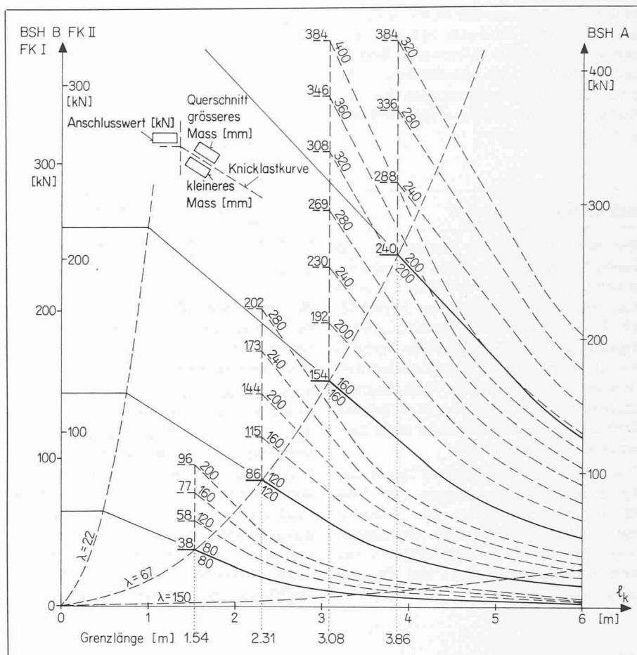
Bild 25. Bemessungsdiagramm für Druck- und Zugdiagonalen mit BSB-Reihenanschlüssen
