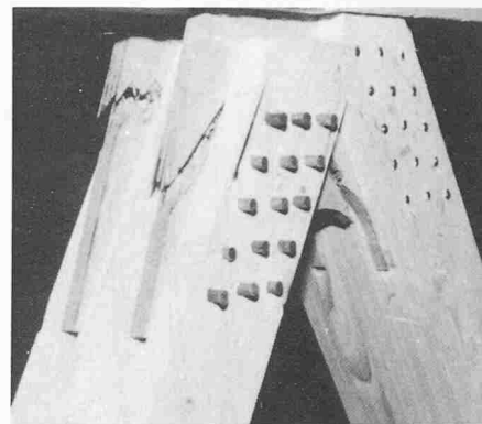
Bild 18. Bruch einer Knotenplatte aus Sperrholz (Verbindungsmitel = Hartholzstifte)
