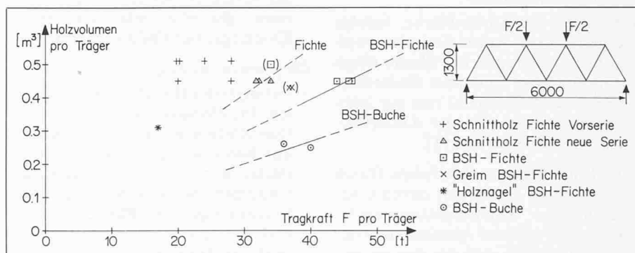
Bild 20. Tragkraft pro m^3 Holzvolumen
