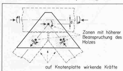
Bild 24. Zonen höherer Beanspruchung
