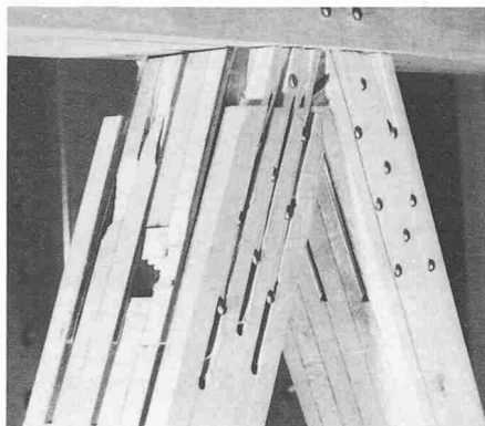
Bild 17. Bruch im Zuganschluss aus Buchen-BSH durch Abscheren des Holzes
