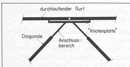
Bild 22. Statische Modellbildung für Knoten
