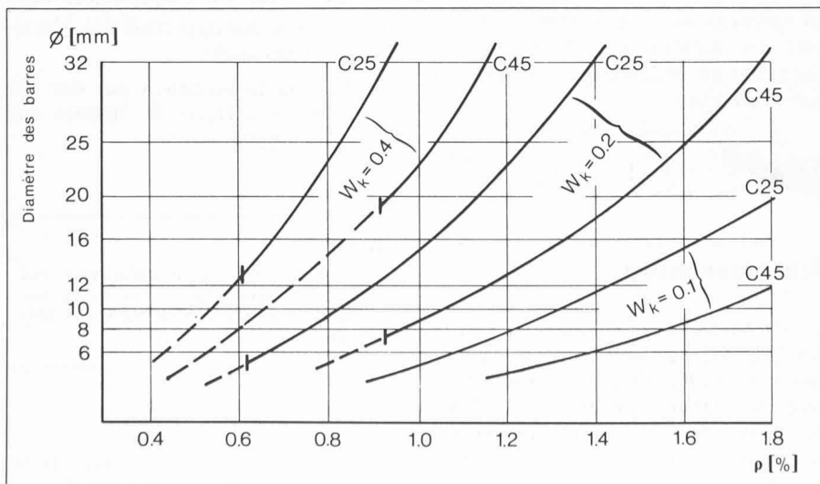
Bild 2. Beispiel eines Diagrammes [3] für die Bemessung des zur Rissebeschränkung erforderlichen Bewehrungsgehalts für mittlige Zugbeanspruchung aus Zwang
