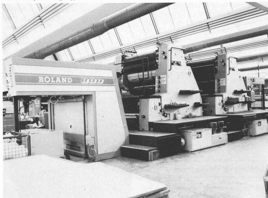
Bild 6. Vierfarben-Bogenoffsetmaschine heute
