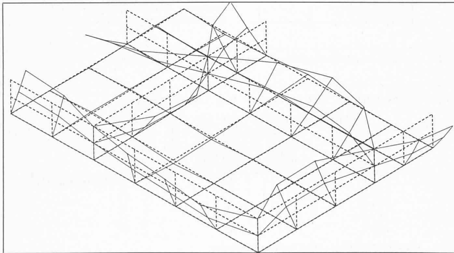
Bild 6. Mit dem Programm Flowers berechnete Eigenschwungsform des gerasterten Oktanten aus Bild 3. Bei dieser Schwingungsform treten in den Wänden starke, in der Decke (bzw. im Boden) schwache Auslenkungen auf
