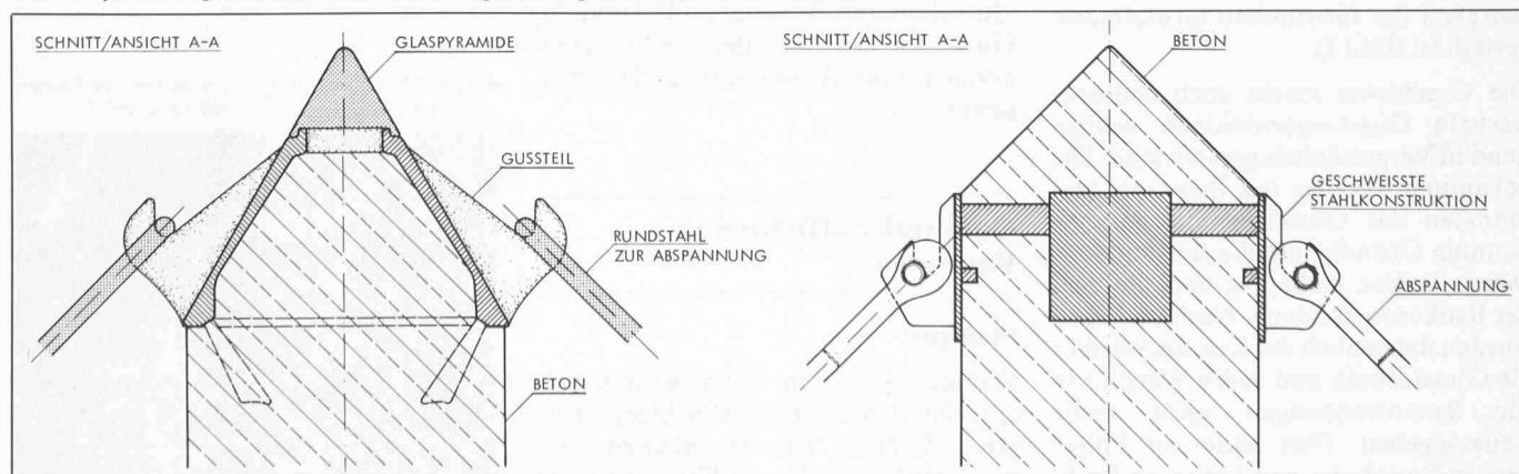
Bild 7. Pylonkronen gemäss Bild 6. Schnitt und Vergleich mit geschweisster Stahlkonstruktion
