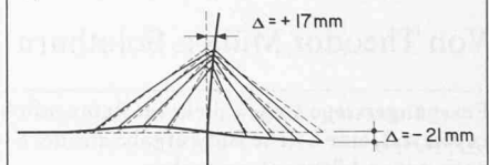
Bild 17. Theoretische Deformationen
