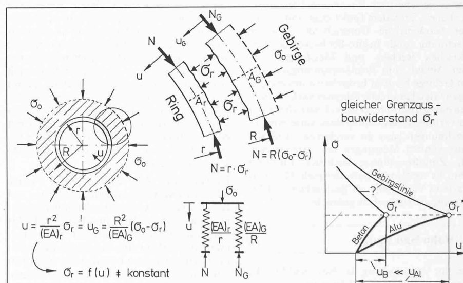
Bild 3. Zur Erklärung des Ausbauwiderstands
