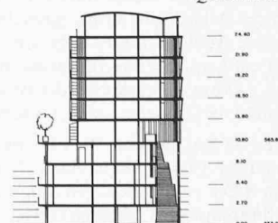
2. Obergeschoss Querschnitt
