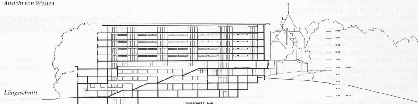
LÄNGSSCHNITT B-B
