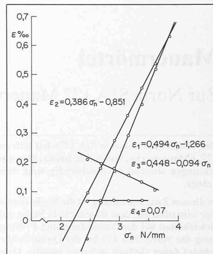
Bild 7. \sigma_n/\epsilon -Diagramm des MBS, 18 cm. Mittelwert aus zwei Versuchskörpern B
