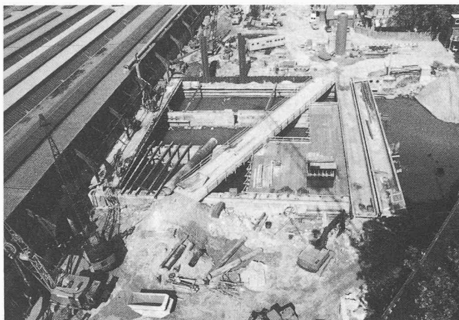
Bild 5. Erste Bauphase der Sihlunterquerung: Die beiden Durchflussöffnungen des Schanzengrabens sind geschlossen (vorne), links entlang der Perronhallen sind die Schlitzwandarbeiten im Gange. Über den drei verbleibenden Durchflussöffnungen sind rechts die beiden verschobenen Gleisbrücken zu erkennen
