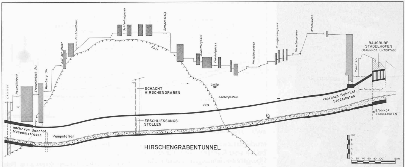
Bild 2. Längensprofil
