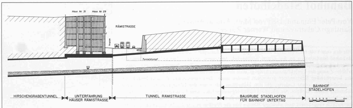
Bild 7. Längsschnitt im Bereich Rämistrasse
