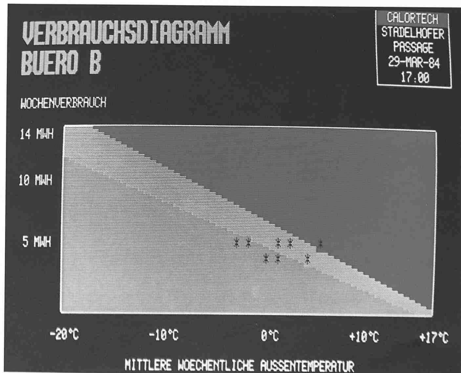
Bild 5. Die (lineare) Beziehung zwischen Wochenverbrauch (z.B. ausgedrückt als Brennerlaufzeit, Endenergieverbrauch oder Nettoenergieabgabe) und der mittleren wöchentlichen Aussentemperatur, aufgrund von Messungen oder theoretischen Bedarfsberechnungen ermittelt, dient zur Beurteilung der Wochenverbräuche, im Bild beispielsweise des Verbrauches des Büros B. Der Wert der laufenden Woche wird durch regelmässiges Blinken gekennzeichnet. Punkte im gelben Sektor entsprechen den Soll-Werten innerhalb eines Bereiches von \pm 10\% , solche im grünen Sektor weisen auf günstige Verbrauchsverhältnisse und solche im roten Sektor auf Unstimmigkeiten hin.
