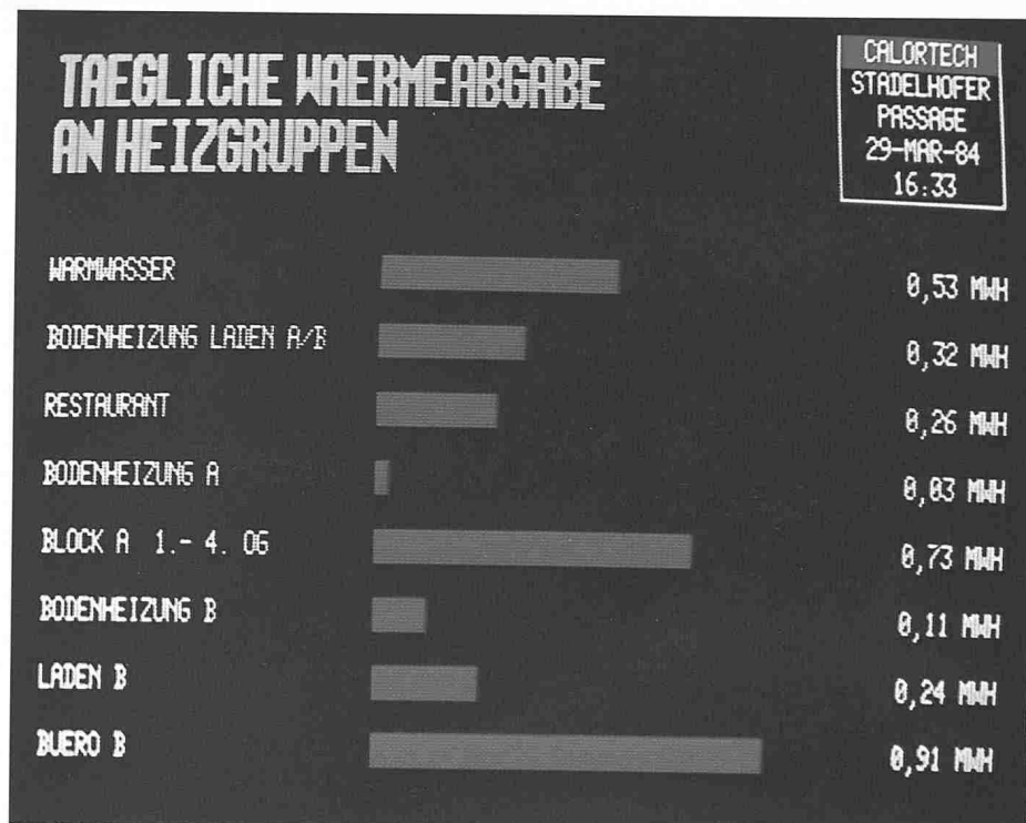
Bild 4. Darstellung (graphisch und numerisch) der Wärmeabgaben der vergangenen 24 Stunden ab 29. März 1984, 16.33 Uhr, für insgesamt 20 Heizgruppen. Rollender Bildschirm und am Ende der 20 Abnehmer zusätzliche Angabe der totalen Wärmeabgabe. Analog liessen sich mühelos auch spezifische Verbrauchszahlen (Energiekennzahlen), Vor- und Rücklauftemperaturen sowie Durchflussmengen aufzeichnen.
