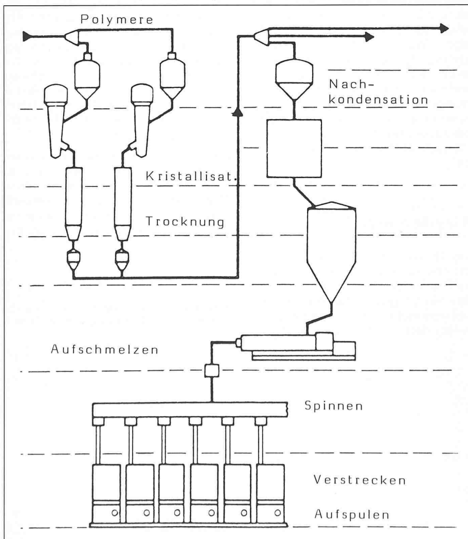
Bild 1. Prinzipschema der Polyester-Spinnanlage
