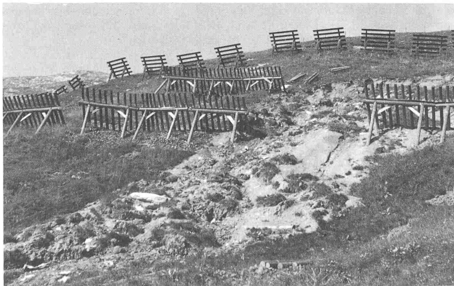
Bild 3 (rechts). Schneebrücken mit nicht aufgefüllter Erdkorberverankerung
