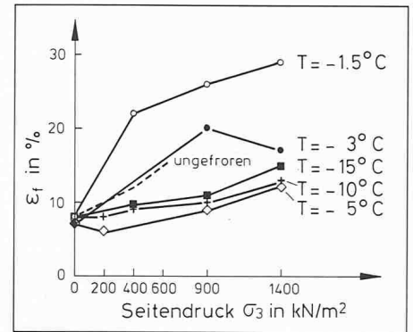
Bild 2. Verlauf der Bruchdeformation in Funktion des Seitendrucks und der Temperatur
