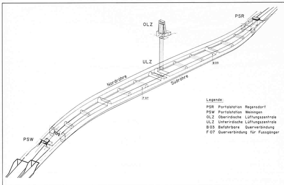
Bild 1. Übersicht Gubristunnel
