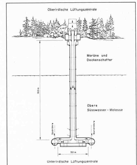
Bild 4. Lüftungsschacht Regensdorf
