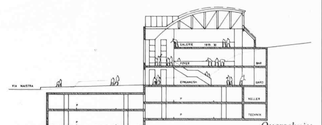
Querschnitt
