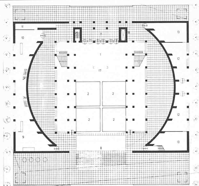
Grundriss Eingangsgeschoß (Mehrzwecksaal/Freilichttheater)
