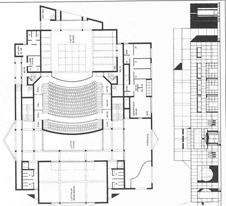
Grundriss Obergeschoss
