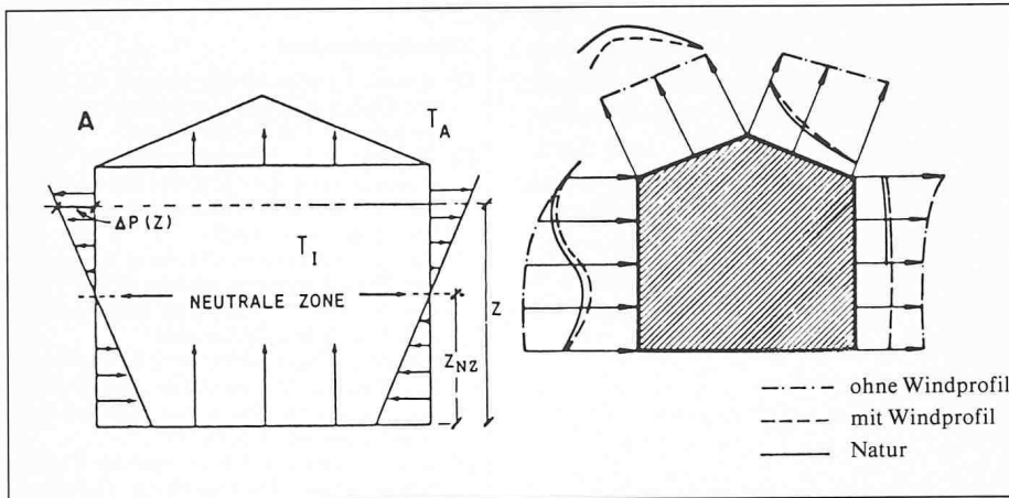
Bild 1. Thermischer Auftrieb und Winddruck
