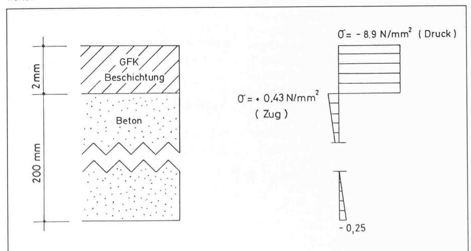
Bild 8. Spannungsverteilung infolge \Delta T = +25^\circ\text{C} in der GFK-Beschichtung und im Beton für eine Schichtstärke des Polyesters von 2 mm und einer Betonstärke von 200 mm mit vorgegebenen Materialkennwerten
