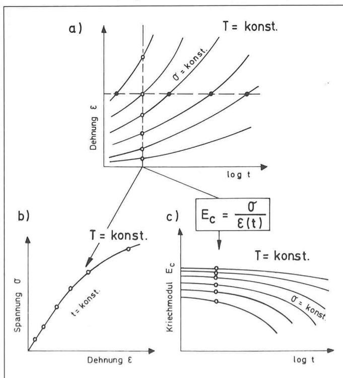
Bild 1. a) Zeit-Dehnlinsen-Diagramm b) Isochrones Spannungs-Dehnungs-Diagramm. c) Kriechmodullinien: E_c(t) = \sigma_0 / \varepsilon(t) . Bild b) und c) können aus dem Zeit-Dehnlinsen-Diagramm ermittelt werden
