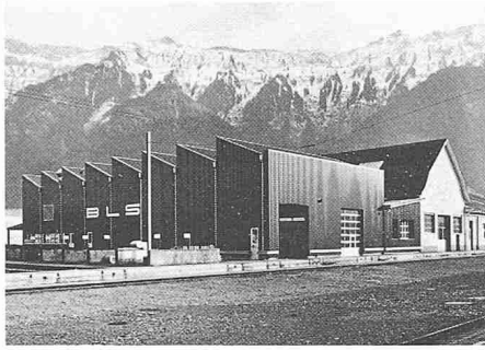
BLS-Werkstätte Bönigen Fahrzeugspritz- und Radsatz-Aufarbeitungshalle 1983; Projekt und Arch.: Reinhard, Bern; Ingenieur: Messerli, Bern
