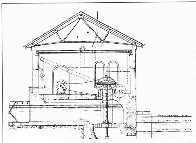
Turbinenanlage à 110 PS Leistung
