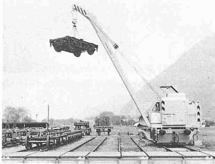
Bern-Lötschberg-Simplon-Bahn BLS 10-t-Eisenbahn-Transportwagen für den Fahrleistungsunterhalt. Projekt und Ausführung: BLS-Zugförderungs- und Werkstättendienst, 1968
