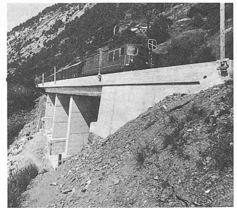
Lehnbauviadukt Hochtenn-Ausserberg Der Ausbau auf Doppelspur talseits vom bestehenden Geleise verlangte auf einzelnen Teilstrecken grösstenteils Lehnbauwerke.
