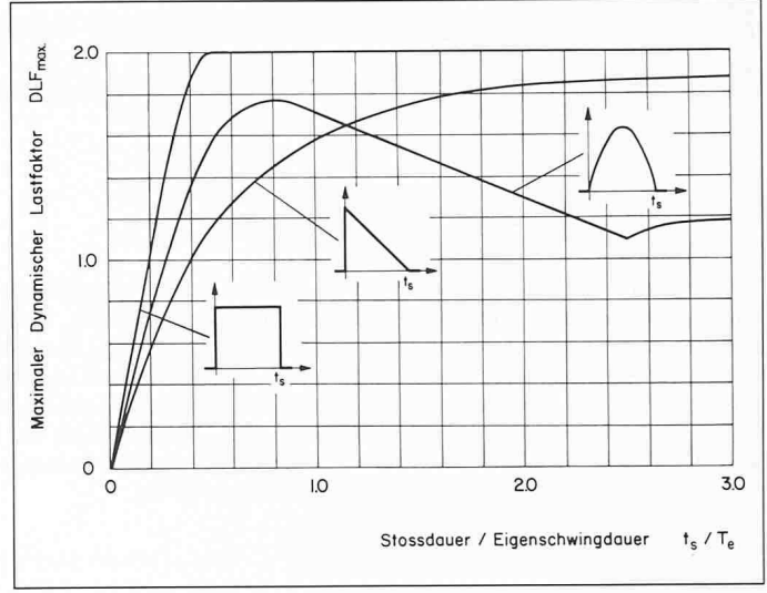
Bild 4. Maximaler Dynamischer Lastfaktor DLF_{max} für den eindimensionalen Schwingen ohne Dämpfung bei Anregung durch Rechteck-, Dreieck- und Halbsinusstoss
