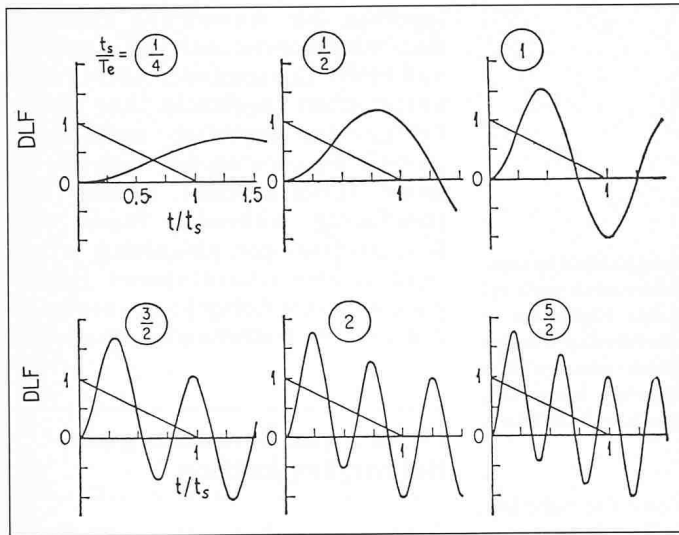
Bild 3. Zeit-Stossantwortkurven für Schwingen mit verschiedenen Eigenschwingungszeiten T_e , angeregt durch Dreieckstoss mit vertikalem Anstieg und Stossdauer t_s [9]
