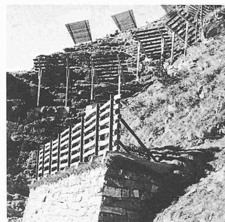
Lawinenverbauungs- und Aufforstungsprojekt Niesen. Beispiel für Entwicklung der Werktypen: 30er Jahre Trockenmauern aus am Ort gewonnenen Steinen; 40er/50er Jahre Erhöhung mit Schneehag aus Eisenbahnschienen und Holzdruckrost (unten); ab 60er Jahre Schneebrücken aus Stahl (mitte); Kolktafeln zur Vermeidung der Gwächtenbildung (Foto: W. Schwarz)
