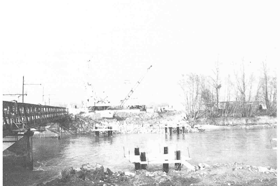
Bild 3. Provisorische Fundationen
