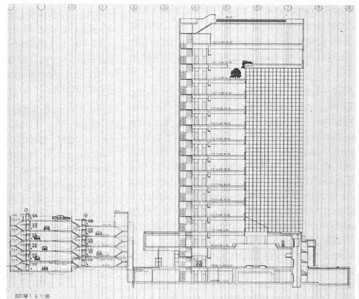
Bild 22. Projektquerschnitt durch ein Bankgebäude
