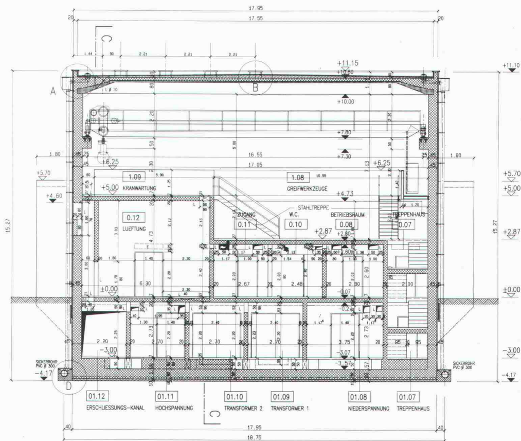
SCHNITT B-B
