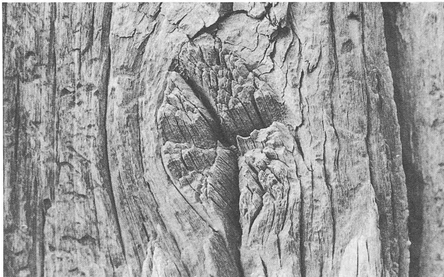
Eichenholz, Türpfosten des Vielzweckhauses aus Uesslingen, Thurgau. Dieses Bauernhaus aus dem 17. Jahrhundert steht heute im Freilichtmuseum Ballenberg
