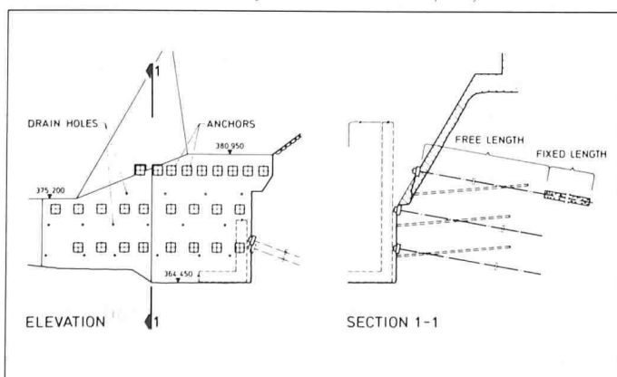
Bild 13 (rechts und unten). Verankerte Stützwand zur Stabilisierung des Felses hinter der Turbinenhalle des Kraftwerkes Derbendikhan (Irak)
