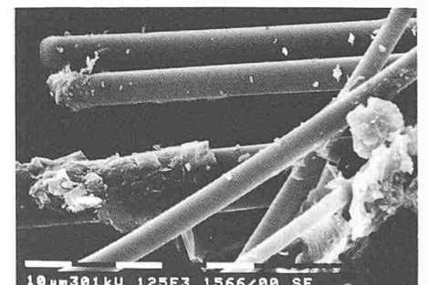
Bild 4. Glasfasern: Im Gegensatz zu Asbestfasern findet keine longitudinale Aufspaltung statt. Die einzelnen Fasern haben zudem einen wesentlich grösseren Querschnitt. Vergrößerung 1250 mal. (Quelle: SUVA)
