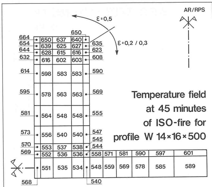
Bild 5. Berechnetes Temperaturfeld im Stahlprofil W 14×16×500
