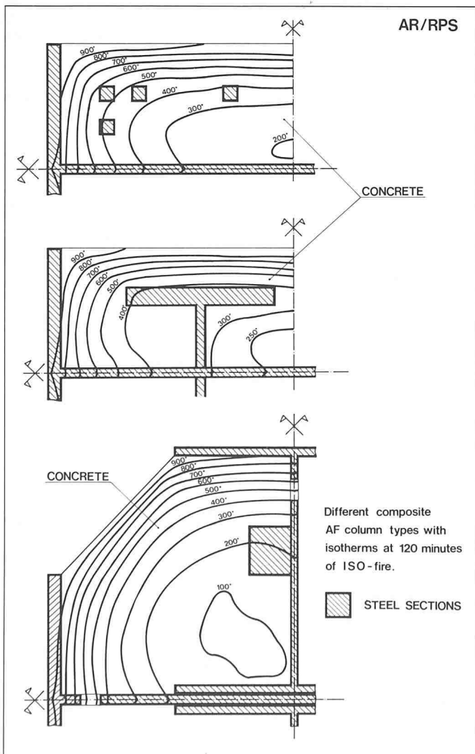
Bild 10. Temperaturverlauf über verschiedene Stützenquerschnitte
