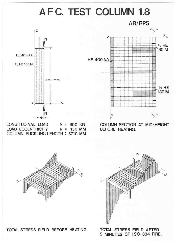
Bild 11 (oben und unten). Exzentrisch belastete Stütze mit internem Spannungsverlauf
