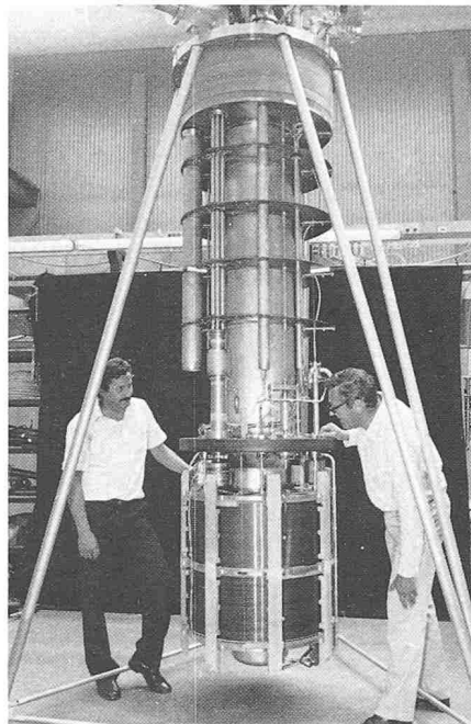
Die Hochfeld-Magnetprobungsanlage HOMER ohne Kryostat. Im unteren Teil des Bildes ist die Niob-Titan-Spule für das Hintergrundfeld von 8 Tesla zu sehen.
