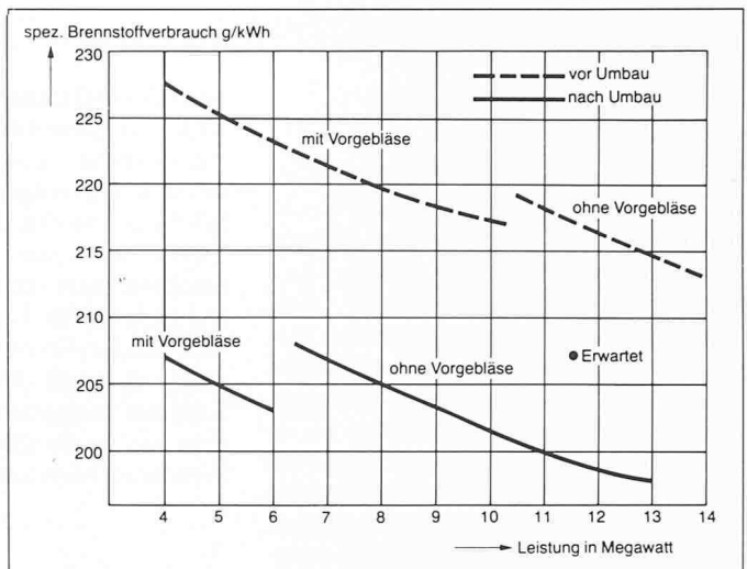
Bild 1. Vergleich des Brennstoffverbrauchs vor und nach dem Einbau neuer BBC-Turbolader
