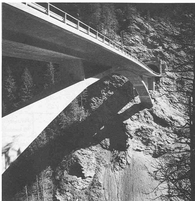
Bild 5. Viamalabrücke
