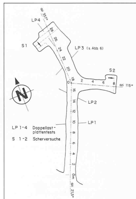
Bild 2. Situation des rund 30 m langen Sondierstollens im Bereich der geplanten Staumauer KW Mulin in der Glennerschlucht
