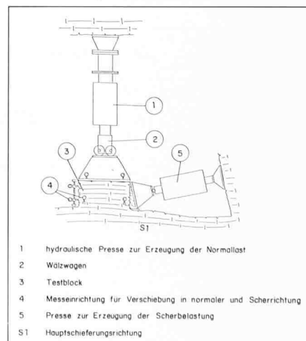
Bild 4. Prinzipskizze des Scherversuchs in situ
