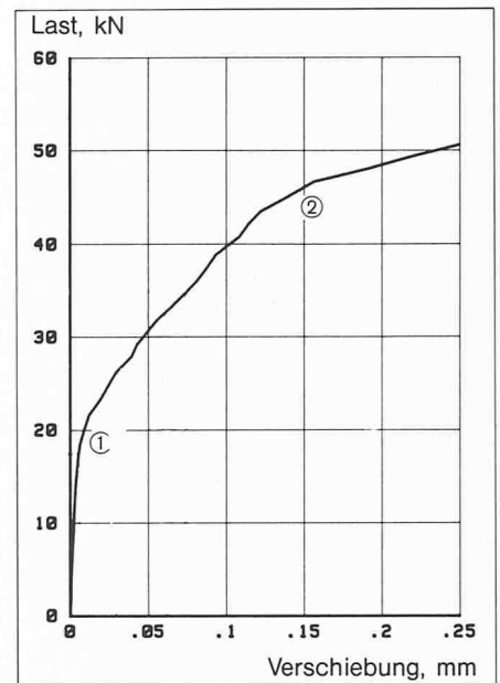
Bild 5. Last-Verschiebungskurve HSL M16, vergrößerter Ausschnitt
