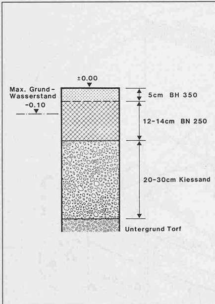
Bild 6. Kantonstrasse Höri-Riet (ZH); Untergrund und Strassenoberbau
