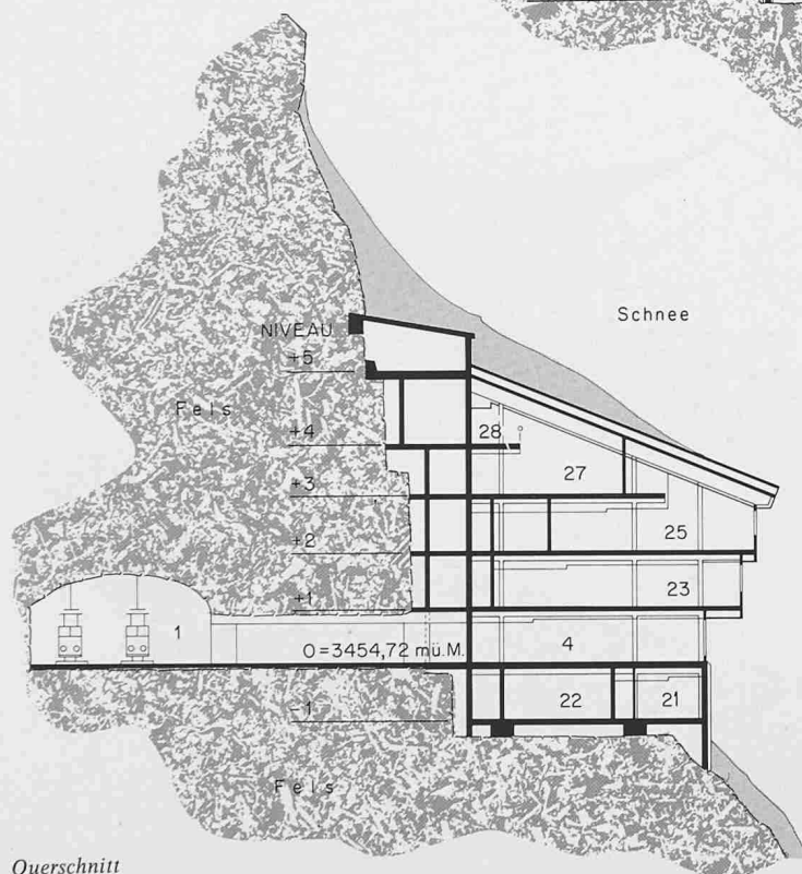
Querschnitt
