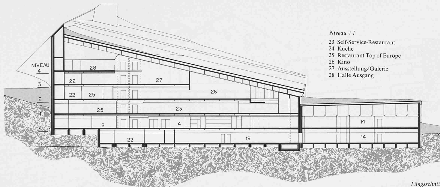
Längsschnitt
