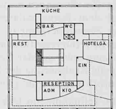
1. Obergeschoss
