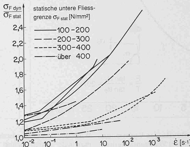
Bild 2. Variation der unteren Fließgrenze für einachsigen Zug oder Druck in Abhängigkeit der Dehnungsgeschwindigkeit aus verschiedenen Quellen nach [4]
