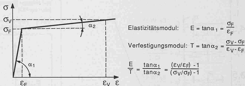
Bild 1. Näherungsweise Beschreibung des Materialverhaltens durch eine bilineare \sigma - \epsilon -Beziehung nach [3]
