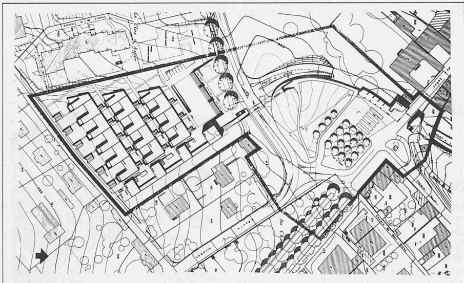
Plan d'implantation 1:3000
