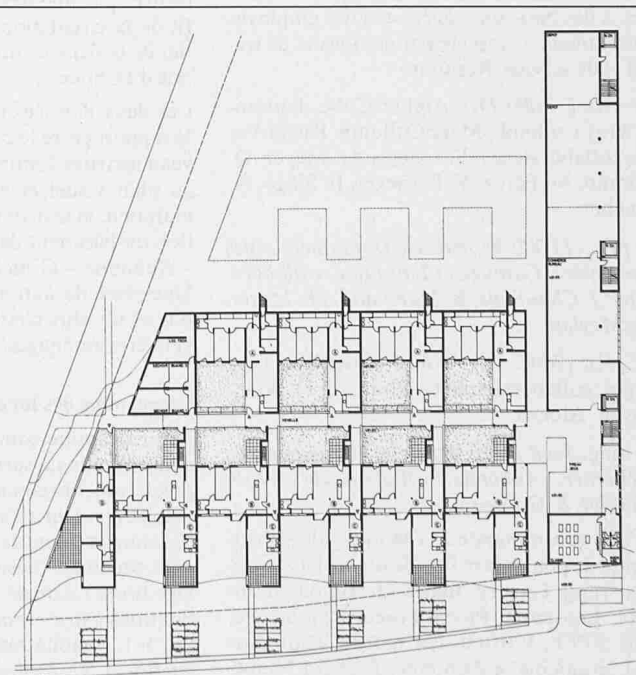
Plan niveau 2, 491.60
