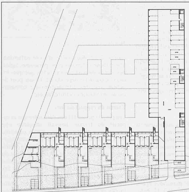
Plan niveau 1, 488.80, 1:1200
