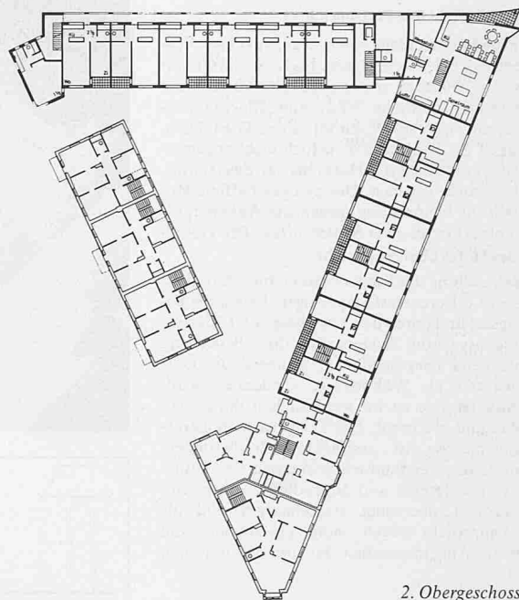
2. Obergeschoss
