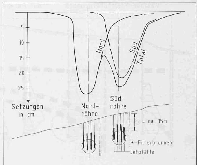
Bild 10. Messquerschnitt mit den grössten Setzungen
