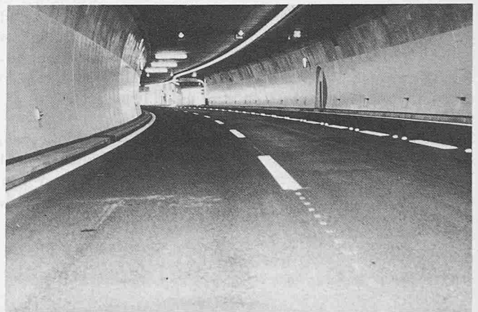
Bild 4. Der dreispurige Milchbucktunnel mit Gegenverkehr
