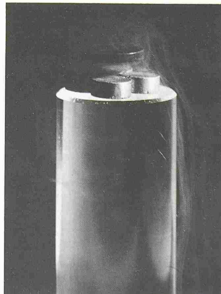
Eine Keramikscheibe schwebt bei ca. 90 K im Magnetfeld von Dauermagneten
