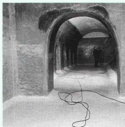
Wasserreservoir Muttengewald: Kombination von verschiedenen Sanierungs-Methoden: Injektionen gegen eindringendes Wasser und zur Verfestigung des Gewölbes, Auskleidung durch starre Abdichtung.
