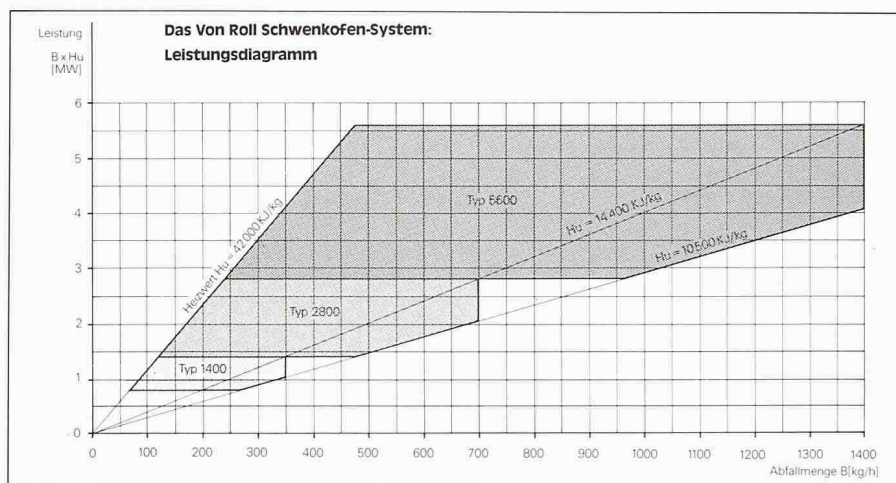
Bild 8. Das Von-Roll-Schwenkofen-System: Leistungsdiagramm
